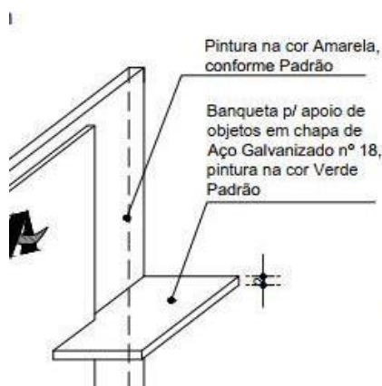
Detalhe da banquetta de apoio em chapa metálica
